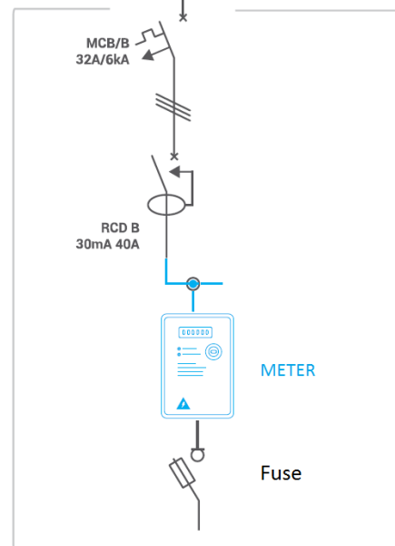
Fig. 13: Schematy wariantów podłączenia 1./2.
