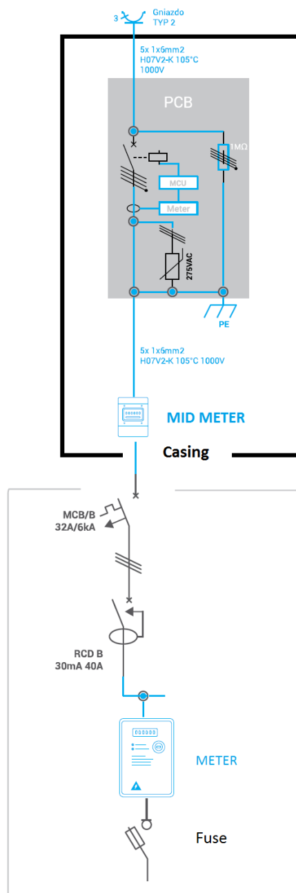
Fig. 14: Schematy wariantów podłączenia 2./2.
