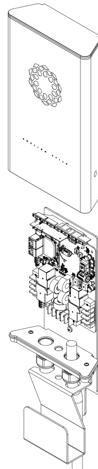
Fig. 4: Fully open Enelion Stilo.
